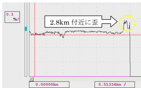
図5 #27 の歪み特性
