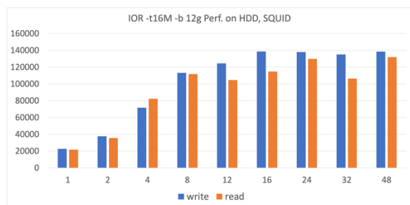
図 8: EXAScaler の HDD 領域での IOR 性能。
