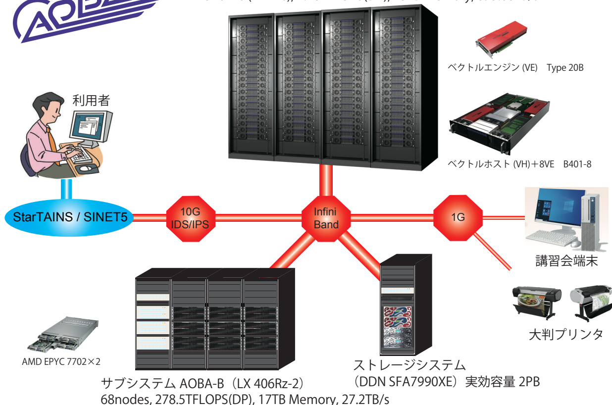
図1 スーパーコンピュータ AOBA の構成
